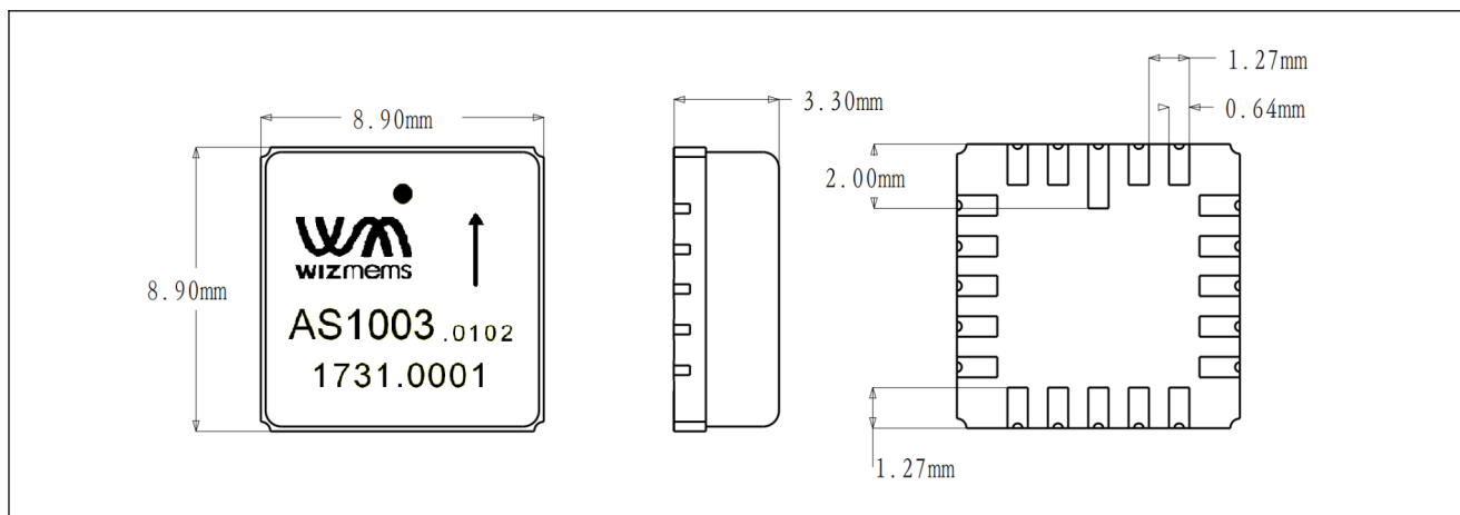
图5. AS1000 封装 (LCC20) 外形尺寸图
