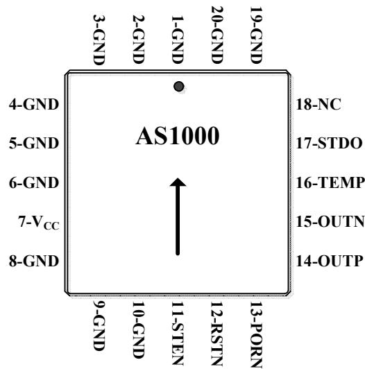
图1. AS1002/AS1003 引脚排布图 ( 顶视 )
