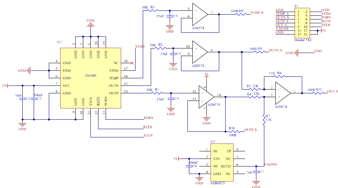
图 4. AS1000 加速度计推荐应用电路
