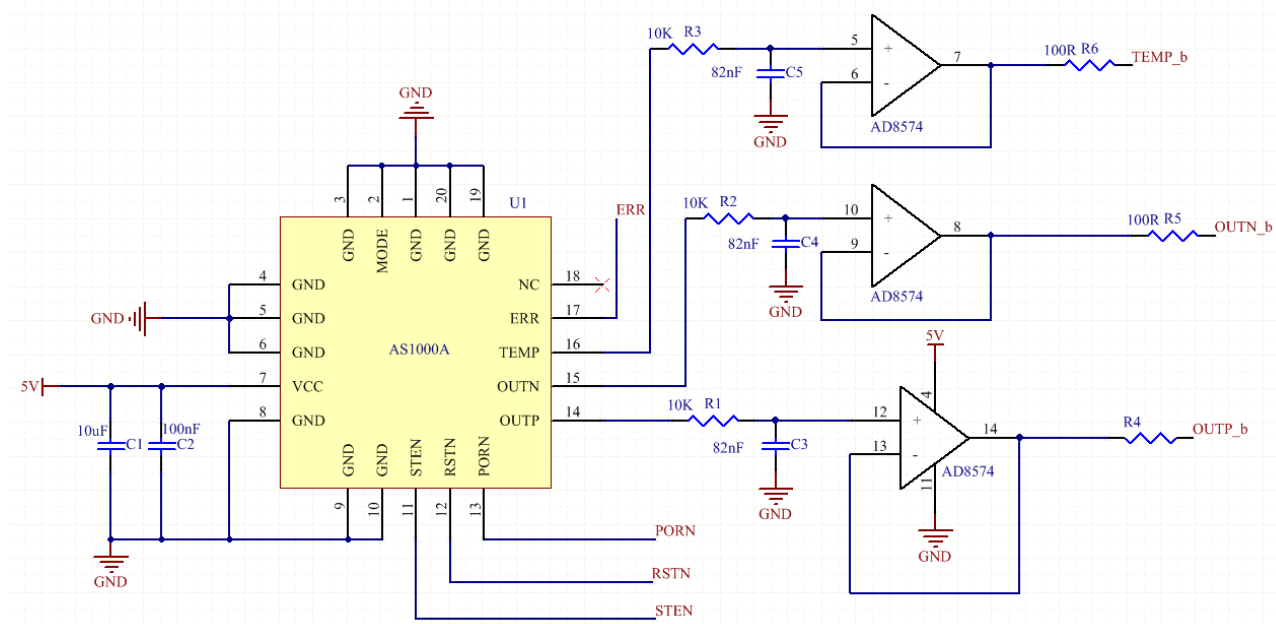
图 5. AS1000A 加速度计推荐应用电路
