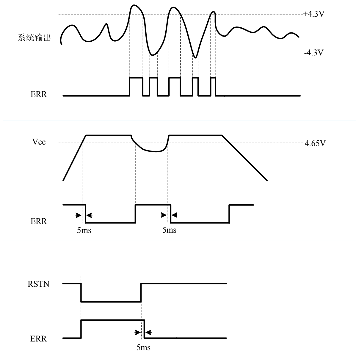
图 3. 系统报错功能示意图
